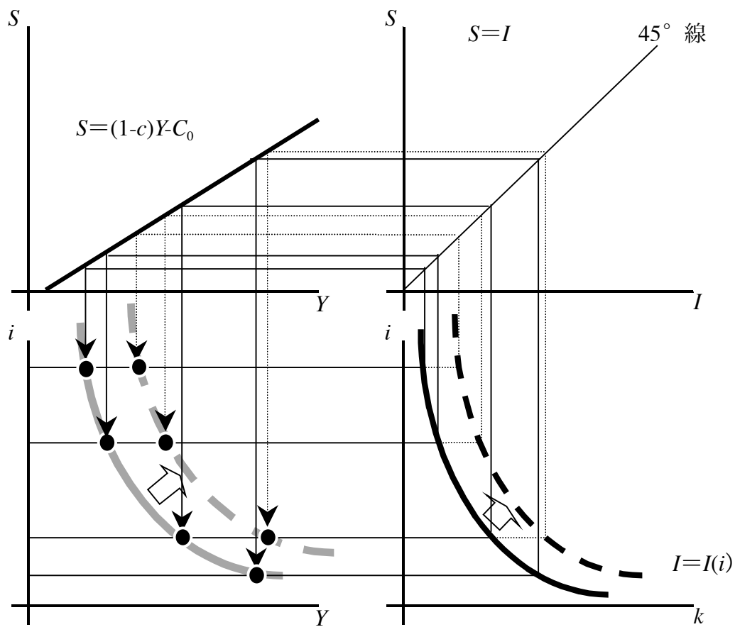
IS 曲線
